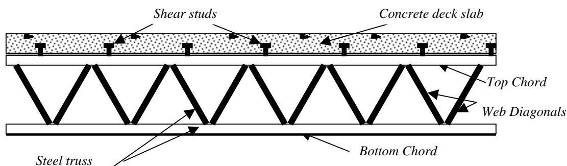
Fig. 6 Composite Truss
